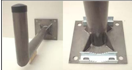
Winkel-Wand-Halter feuerverzinkt mit 4 Knotenblechen und 1 Knotenblech im Schenkel waagrecht/lotrecht Grundplatte 250 x 250 x 5mm 76er Rohr
